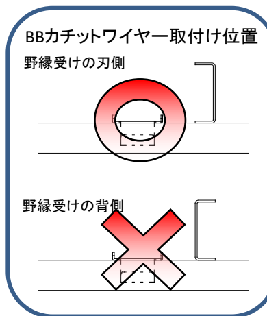
正面図(取付後)
